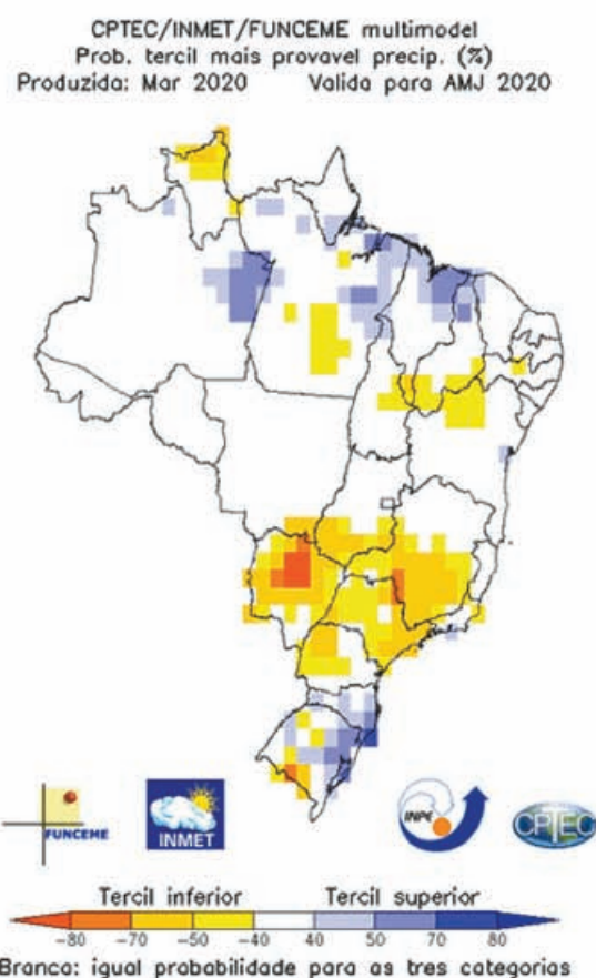
>> Figura 4 - Previsão climática sazonal por tercil (categorias abaixo da faixa normal, dentro da faixa normal e acima da faixa normal) para o trimestre abril, maio e junho. As áreas em branco indicam padrão climatológico (igual probabilidade para as três categorias). Fonte: CPTEC/INPE, INMET e FUNCCEME
