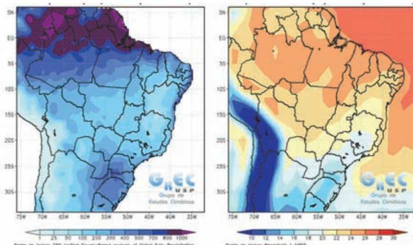
Figura 2 - Climatologia da precipitação (esquerda) e temperatura do ar (direita) do trimestre de abril, maio e junho. Fonte: GrEC/USP.
