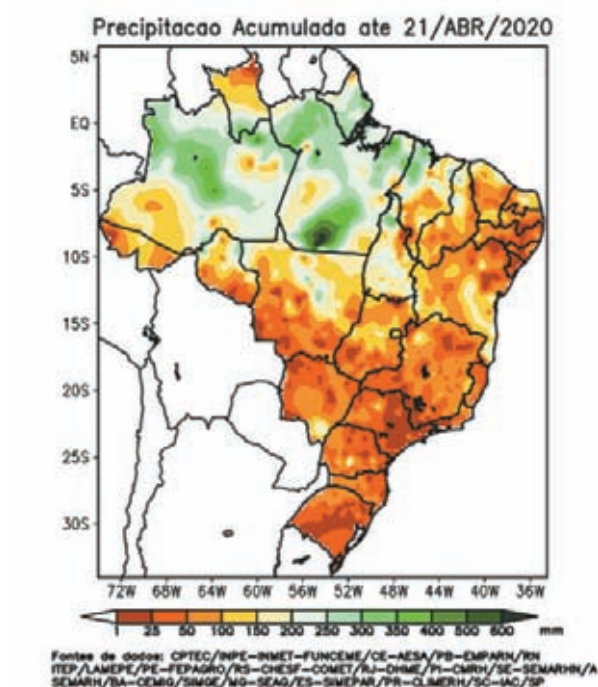
>> Figura 3 - Precipitação acumulada entre os dias 01 a 21 de abril de 2020. Fonte: CPTEC/INPE
